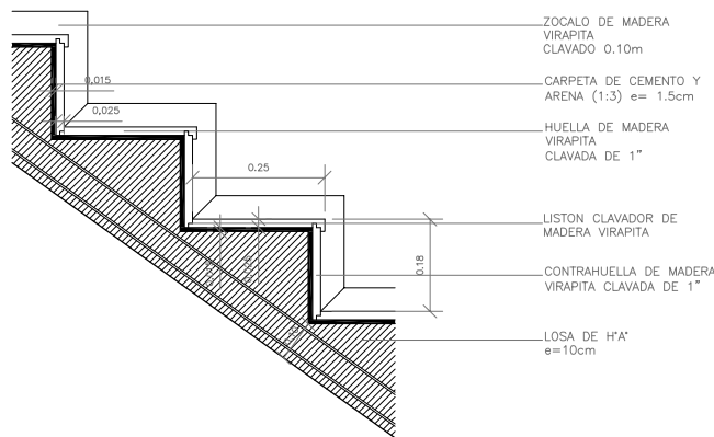
DETALLE ESCALERA 1 Esc. 1:10
