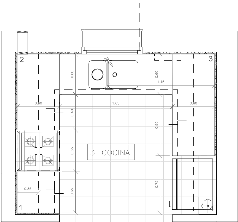
3/COCINA PLANTA COCINA Esc. 1:25
