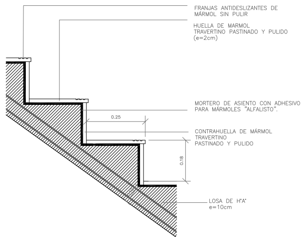
DETALLE ESCALERA 2 Esc. 1:10
