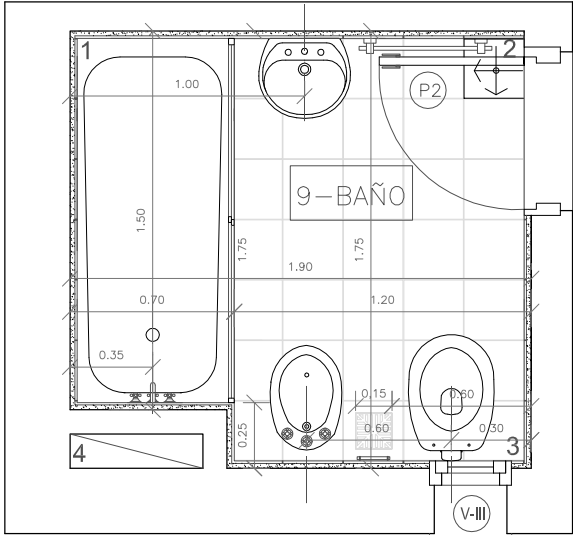
9/BAÑO PLANTA BAÑO Esc. 1:25
